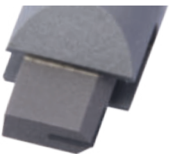
Diamond dresser Rhomboid 3 x 0,4 x 0,4 mm, Total bearing surface 0,48 mm 2 , r = 0,25 mm
