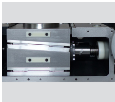
Elektromechanische Richtspaltregelung (patentiert)
