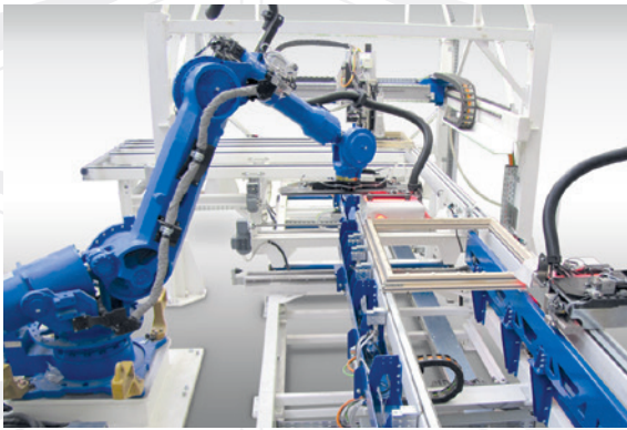
Fensterproduktionsanlage
