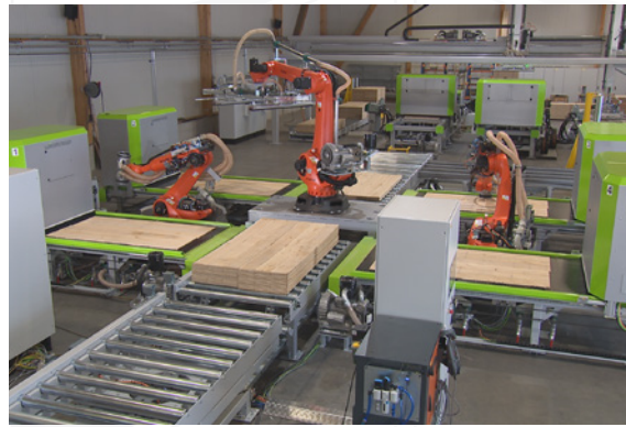
Vollautomatische Reinigung und Ausbesserung von Platten
